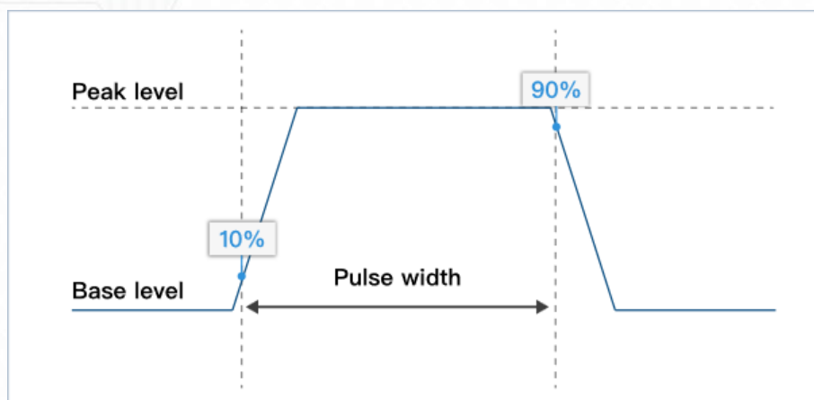
脉冲宽度定义
