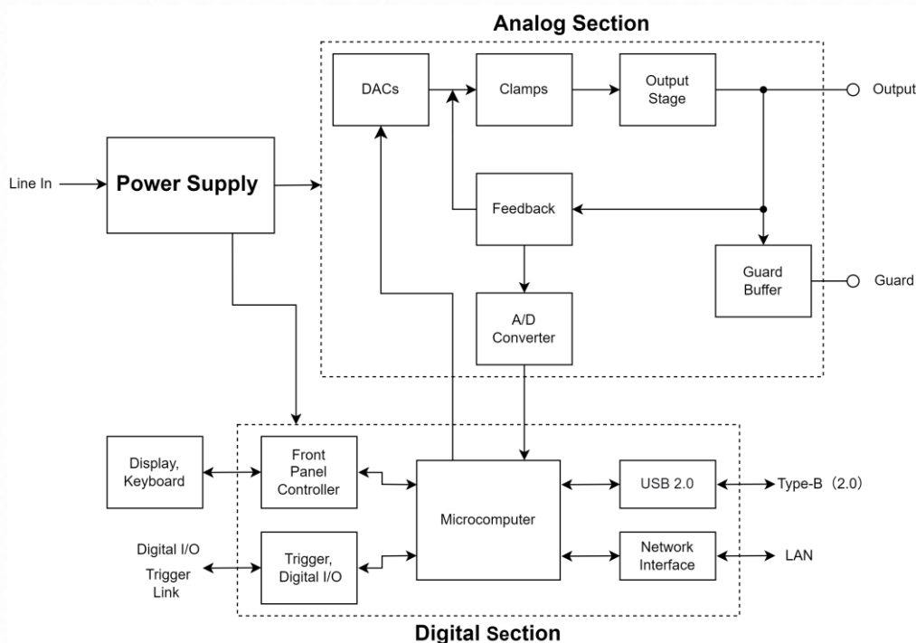
S3012H 架构图
