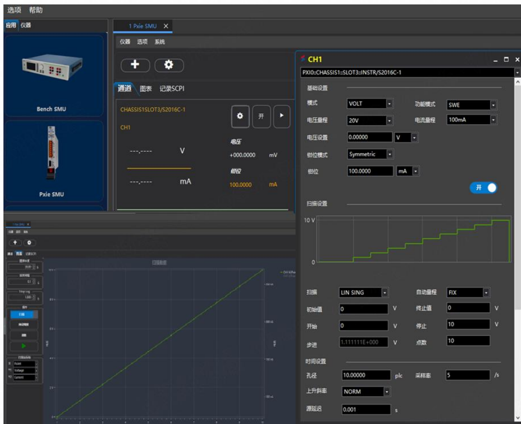
GUI 界面
