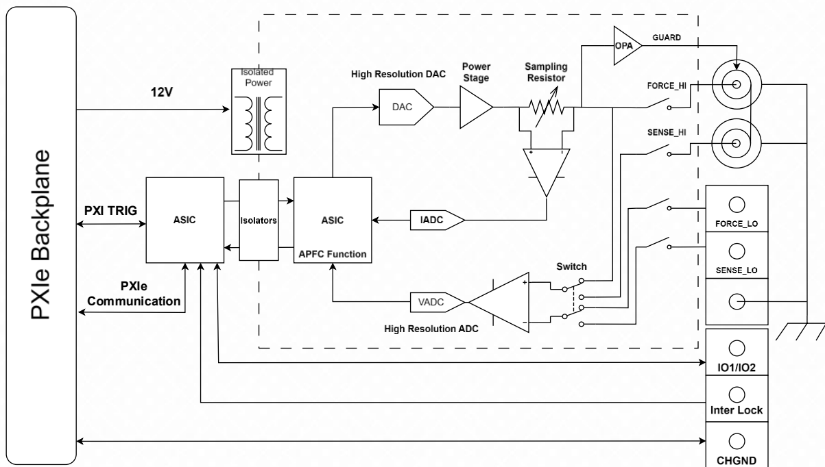
S2016C 架构图
